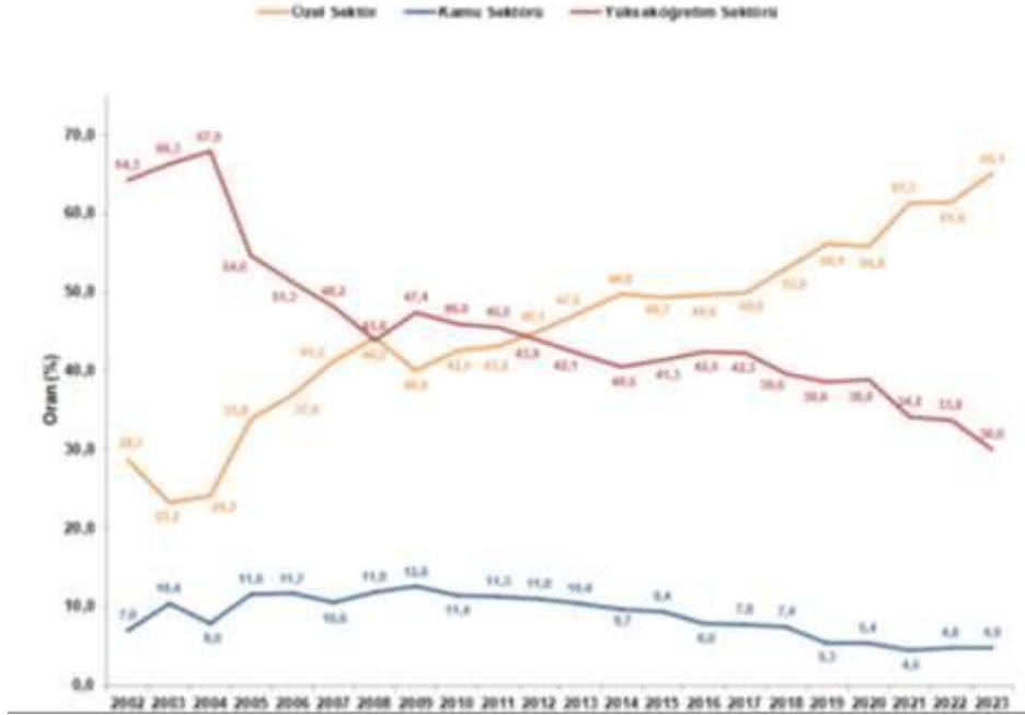
Şekil 6. Gerçekleştiren sektörler bazında Ar-Ge harcamaları oranı (%)
